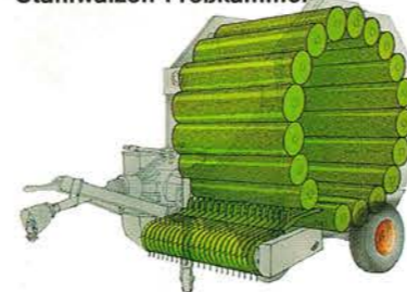
Stahlwalzen-Preßkammer
